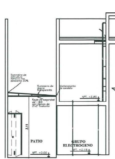
Detalle Estructura en Ducto ESCALA 1:50
